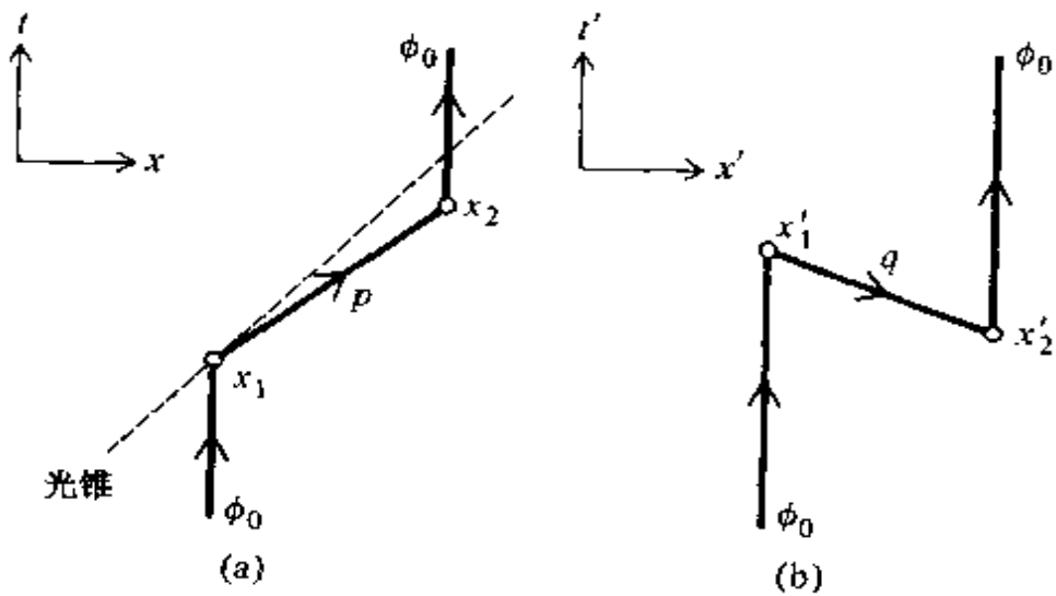
图 2 从两个不同的参照系上来观察同一过程 (a)原参照系( t_2 > t_1 )；(b)动参照系( t'_2 < t'_1 )
