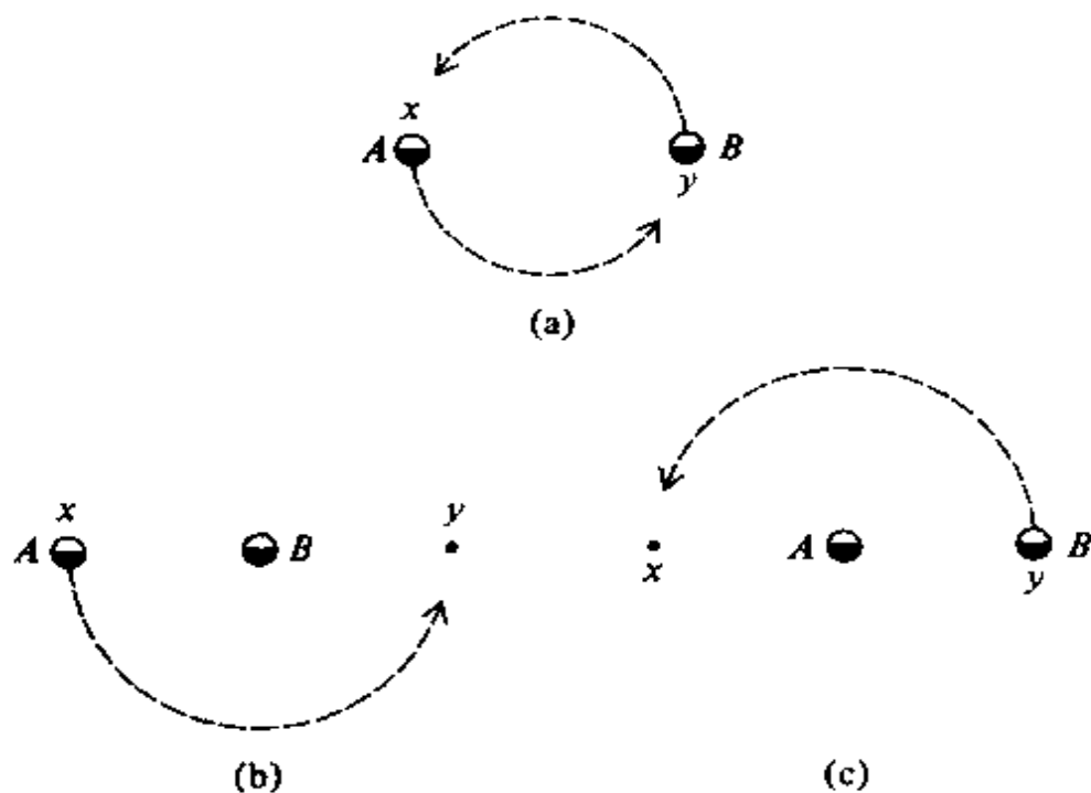
图 15 两组电荷-磁单极间的交换图
