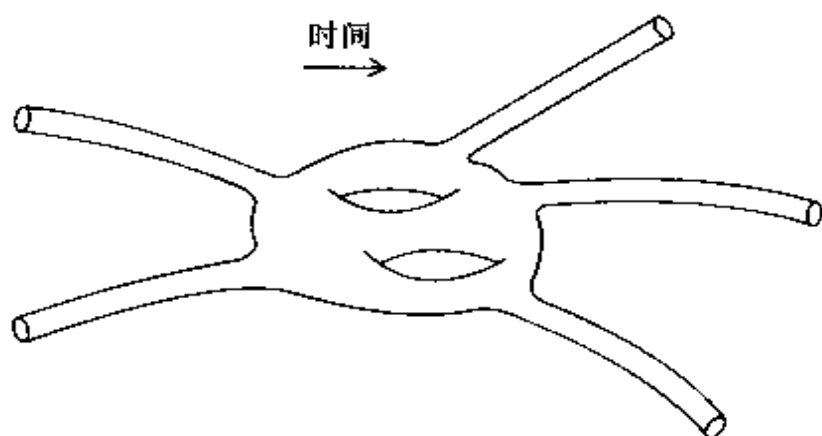
图3 两个粒子变成三个粒子的散射过程
