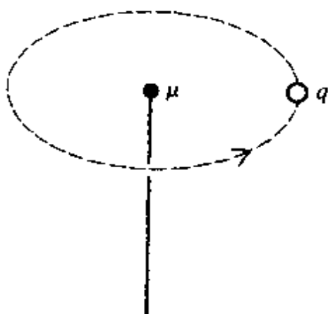
图 14 将电荷 q 绕磁单极转过 360^\circ
