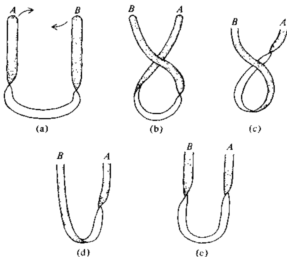
图 16 在(a)至(e)的一系列的图中, 绶带两 endpoints 的位置对调了。注意(e)图右端对着我们的是(a)图中的反面。要使它完全恢复原样, 就需要右边绶带绕垂直轴再转过 360^\circ
