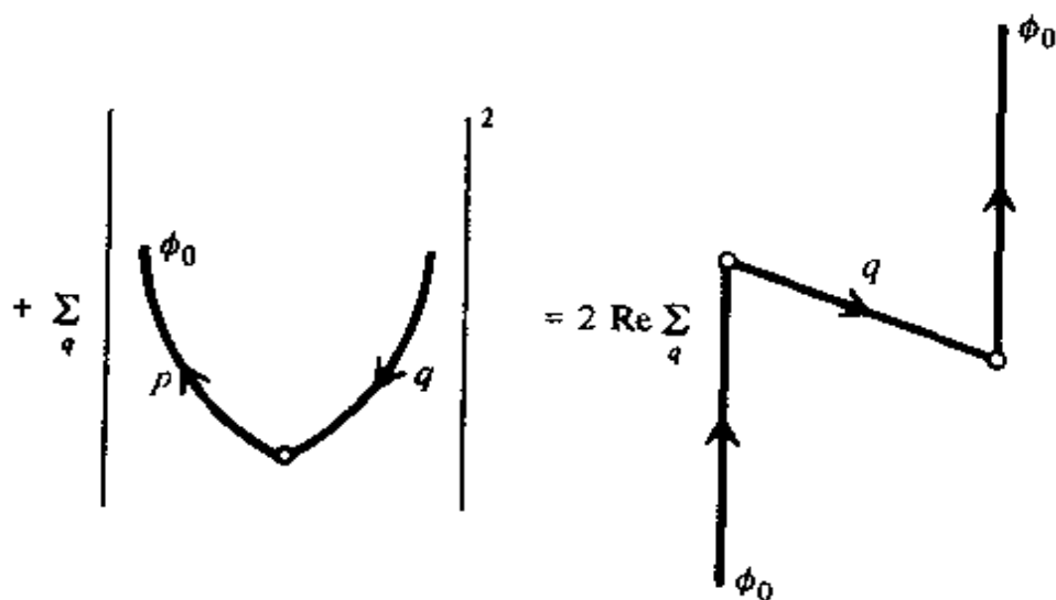
图 10 \frac{1}{2} 自旋粒子与图 4 相当的等式
