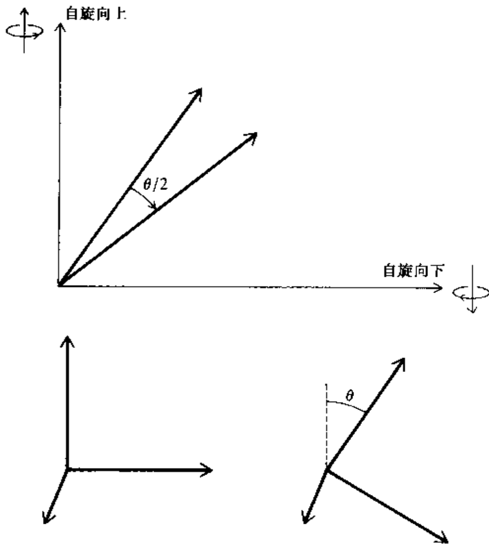
图 2 转动对电子自旋的作用
