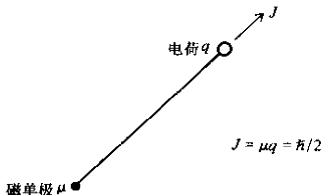
图 13 电荷 q 附近的一个磁单极
