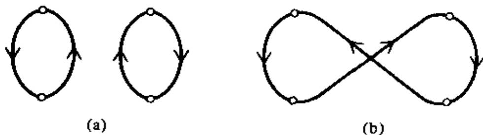
图 9 (a) 无粒子交换时的两对粒子 - 反粒子偶的产生 (b) 有粒子交换时的两对粒子 - 反粒子偶的产生
