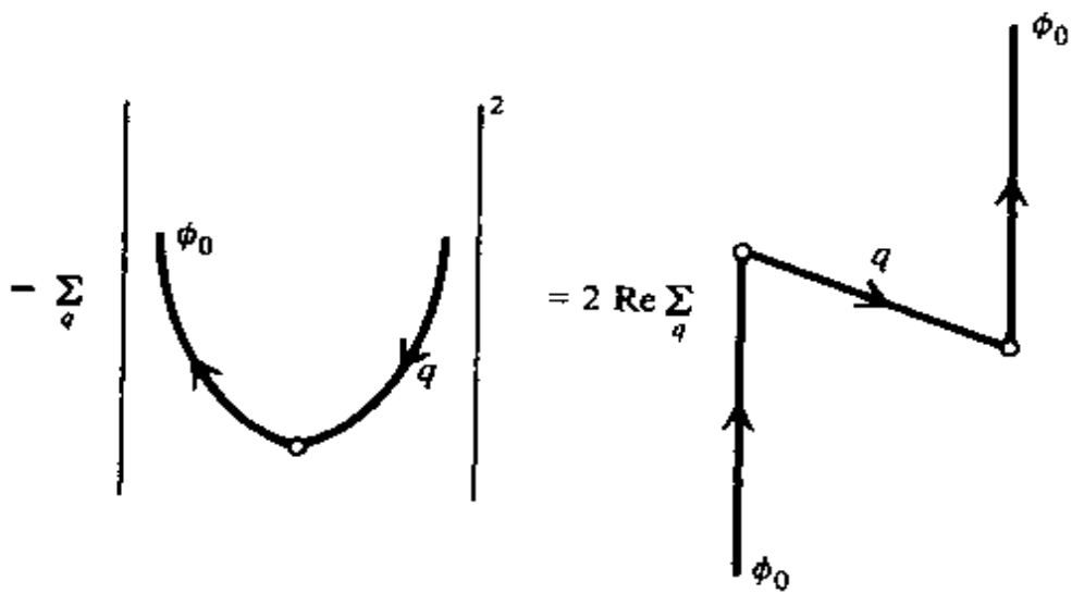
图 4 一个图形等式，其中粒子自旋为 0，图中含有反粒子
