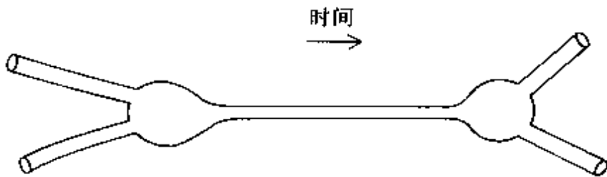
图 4 一根弦的截面，包含着自旋为 2 的无质量粒子的发散和重新吸收
