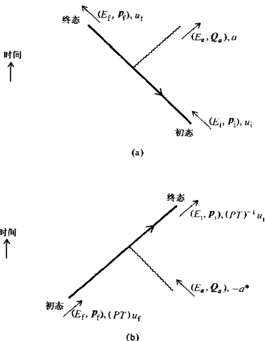
图 11 (a) 一个反粒子发射一个光子的过程 (b) 相应的粒子吸收一个光子的过程
