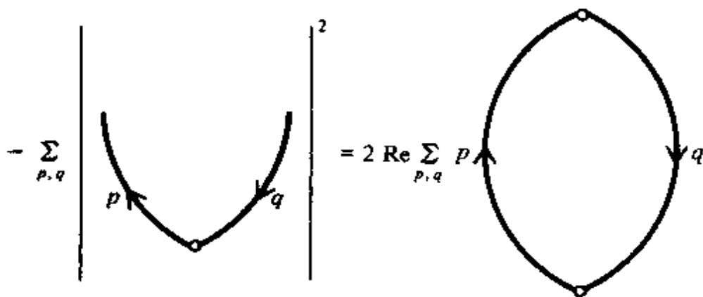
图 6 初态为真空时的一个图形等式
