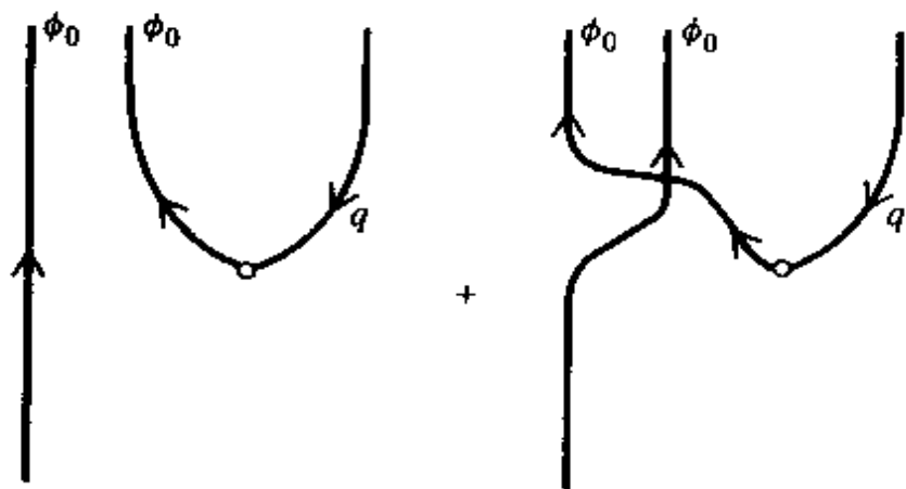
图 8 其中一个图形来自图 7(f), 另一个为其交换图形
