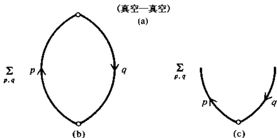
图 5 从“无粒子态”即真空开始的几个(最低阶的)过程
