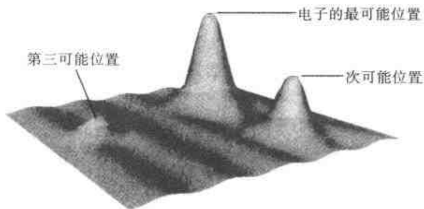
图 4.9 哪里最容易找到电子，哪里的电子波最大；而在波小的地方发现电子的机会也越小。
