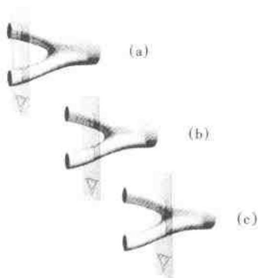
图 6.8 乔治看到的两根弦在相继三个时刻的样子。在(a)和(b)，两根弦越靠近；它们在(c)第一次接触(从他的观点看)。
