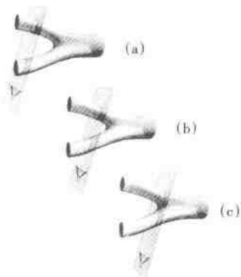
图 6.9 格雷茜看到的两根弦在相继三个时刻的样子。在(a)和(b)，两根弦越靠近；它们在(c)第一次接触(从她的观点看)。
