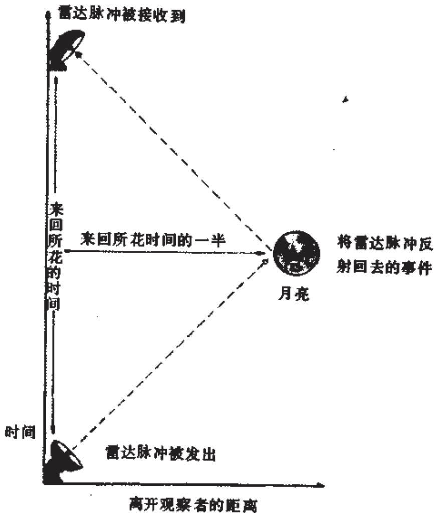
图2.1 时间用垂直坐标测量，离开观察者的距离用水平坐标测量。观察者在空间和时间里的途径用左边的垂线表示。到事件去和从事件来的光线的途径用对角线表示。
