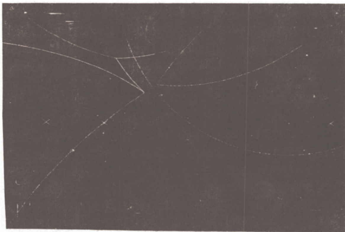
图5.2 一个质子和一个反质子在高能下碰撞，产生了一对几乎自由的夸克。
