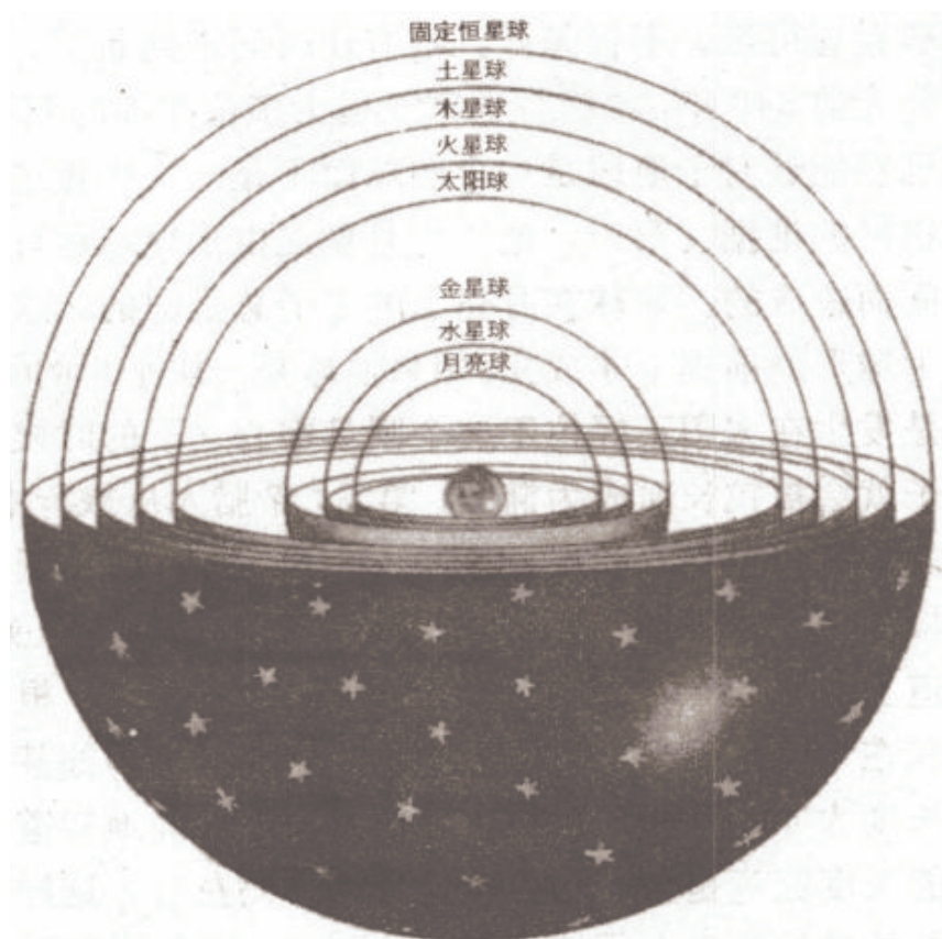
图1.1 从最里面往最外面顺序为月亮球、水星球、金星球、太阳球、火星球、木星球、土星球和固定恒星球。最中心为地球。
