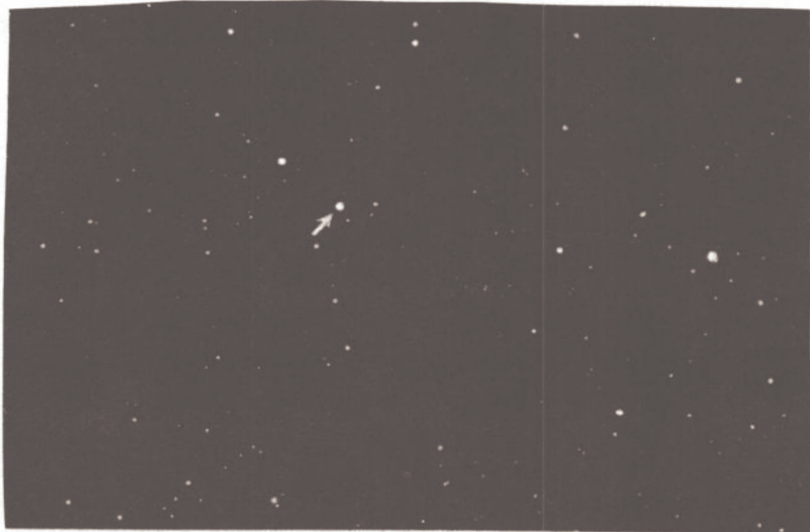
图6.2 在靠近照片中心的两个恒星之中更亮的那颗是天鹅X-1,被认为 是由互相绕着旋转的一个黑洞和一个正常恒星组成。
